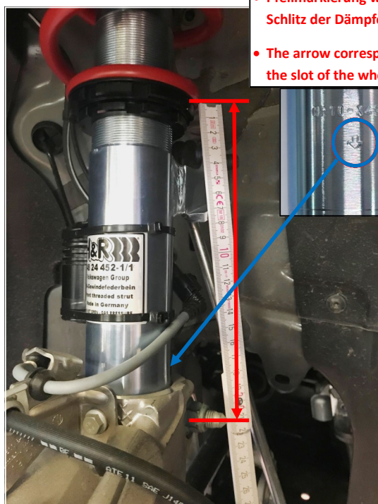
Abb. 4: Einbaulage / Einstellmaß VA (Abb.ähnlich) Fig. 4: FA mounting position / adjustment dimension (Fig. may vary)
